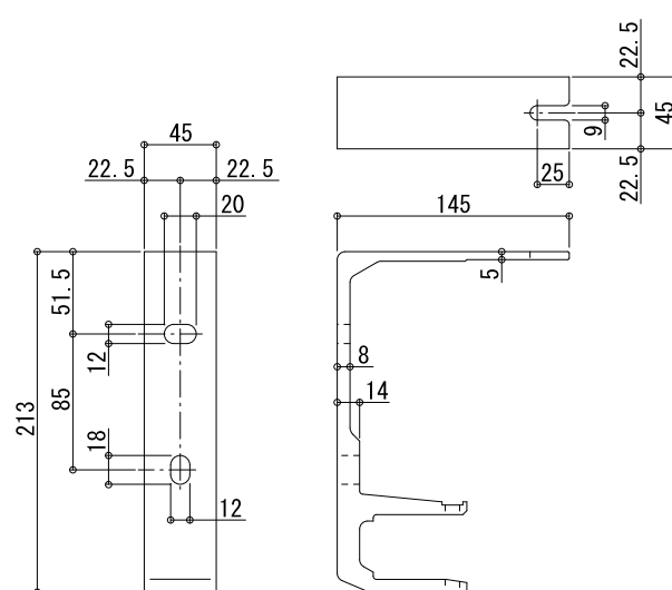
[2] 補助取付ブラケット
