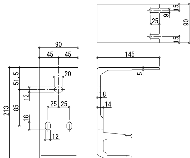
[1] 取付ブラケット
